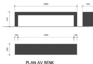
PLAN AV BENK
