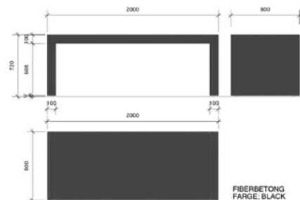
PLAN AV BORD
